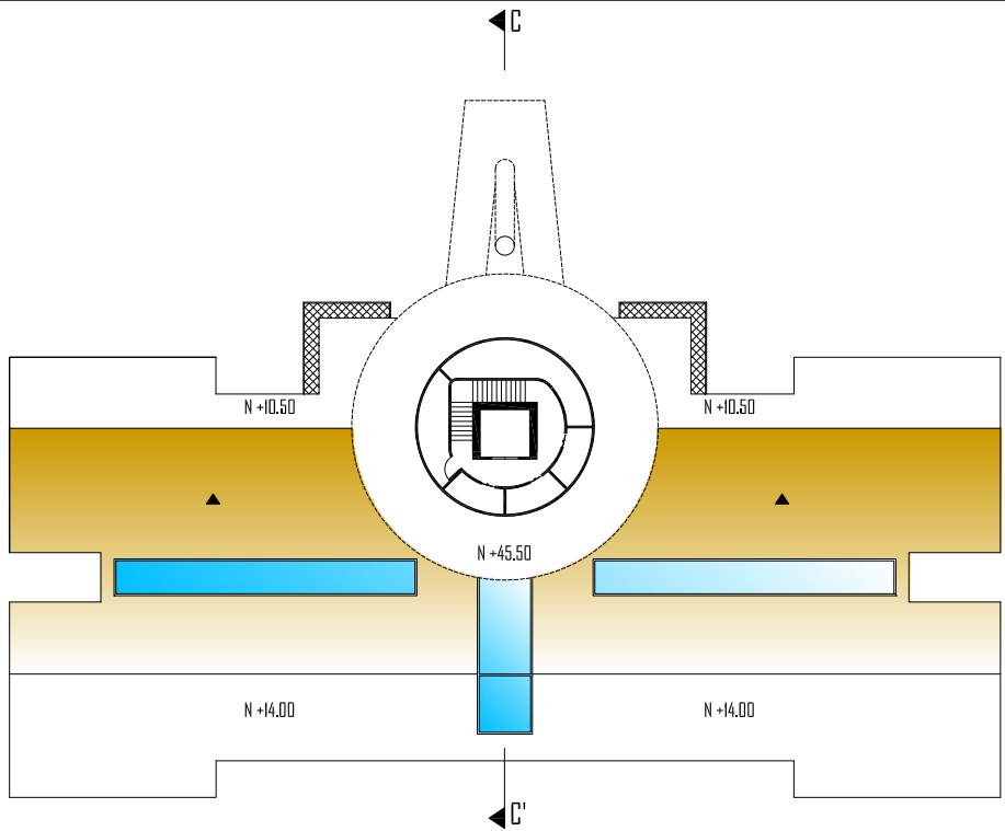
PLANTA NIVEL 43
