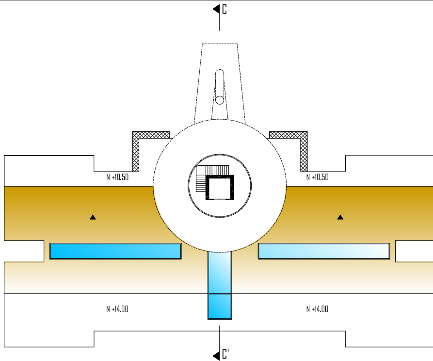
PLANTA NIVEL 45.5
