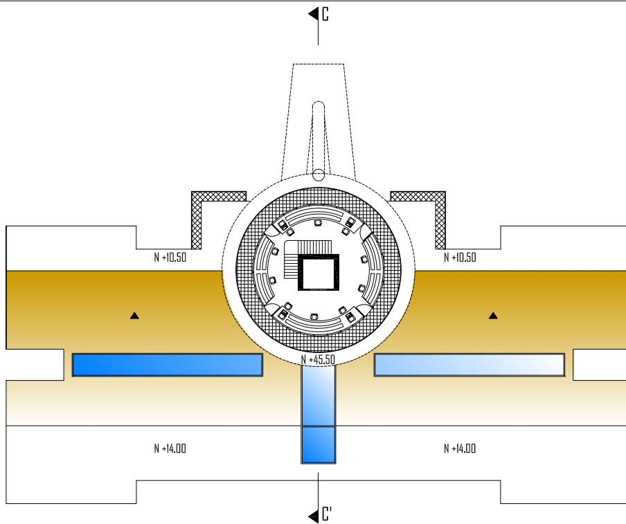
PLANTA NIVEL 52.5
