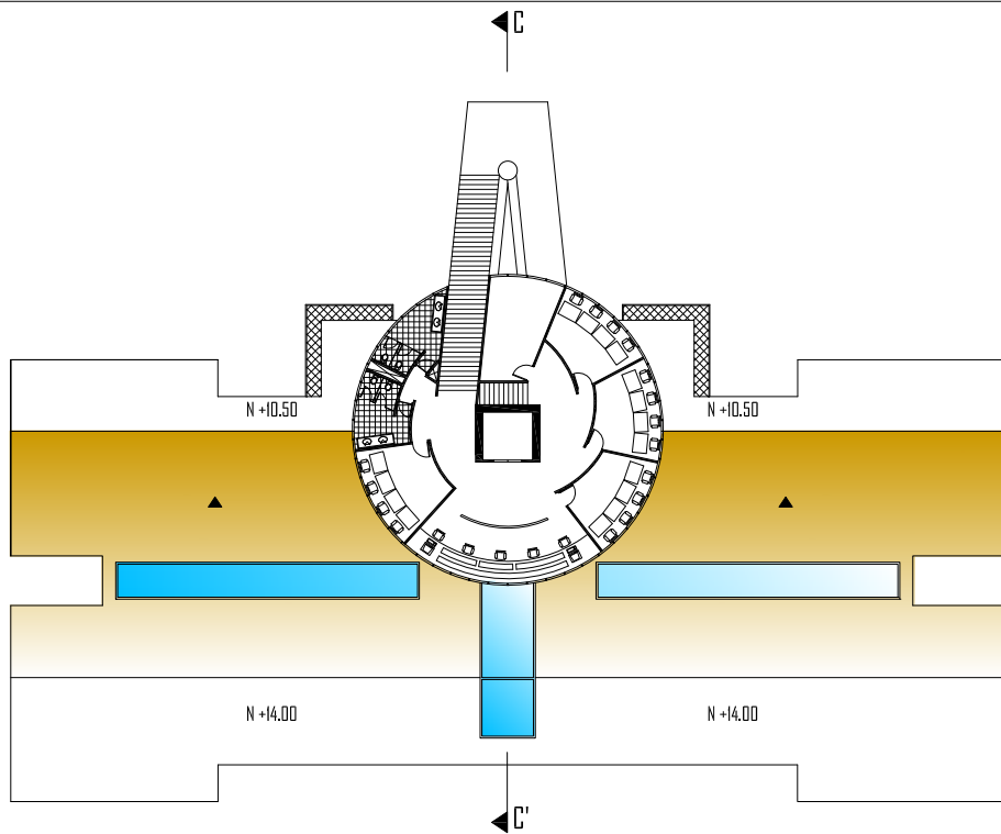
PLANTA NIVEL 42
