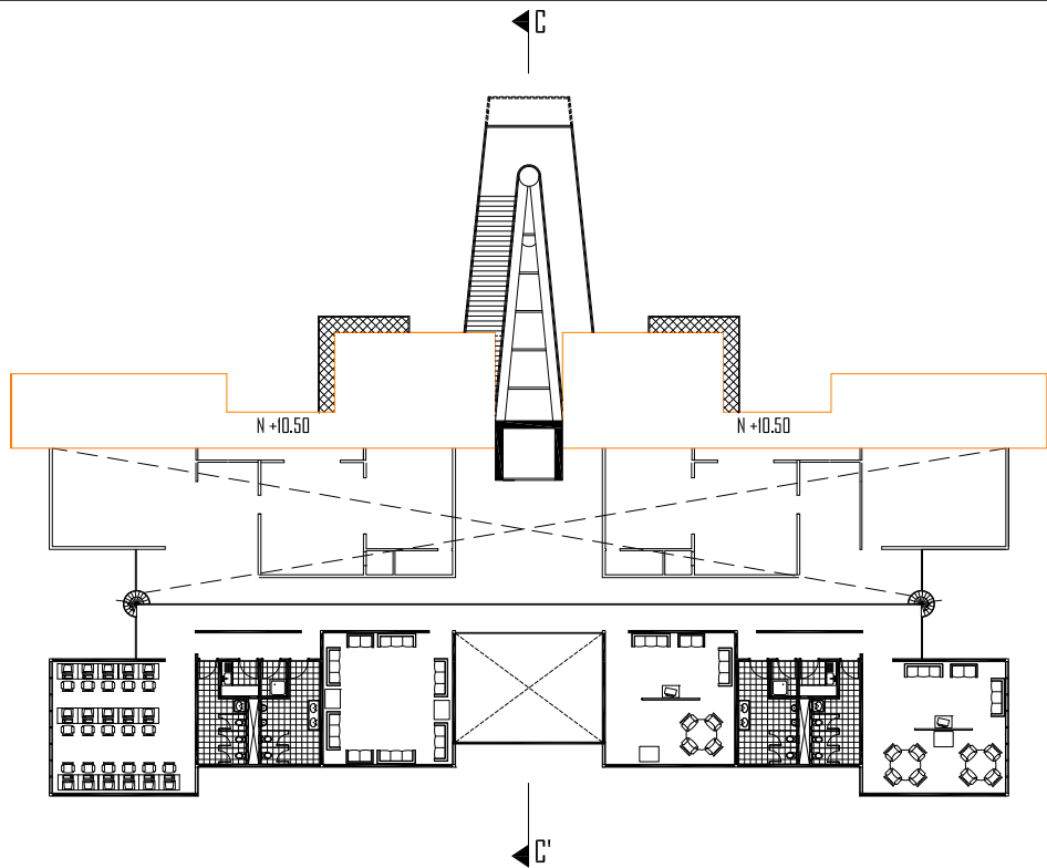
PLANTA NIVEL 10.5
