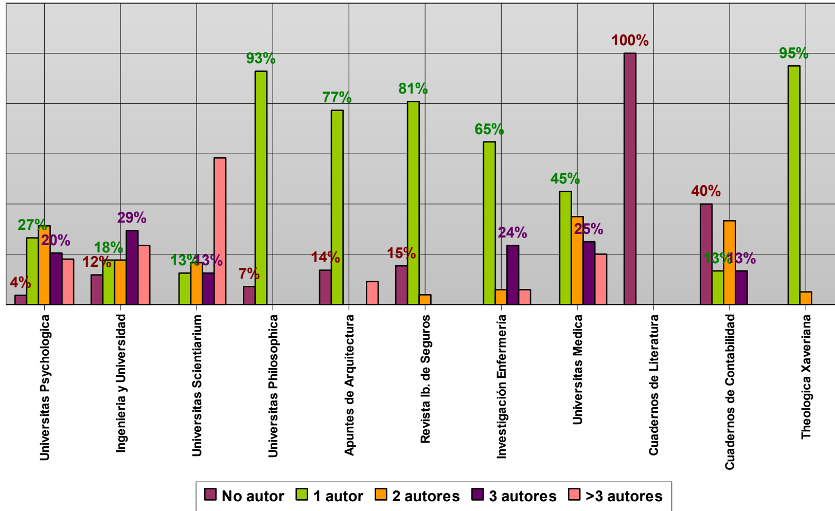
Tratamiento de Artículos Publicados: Número de autores
