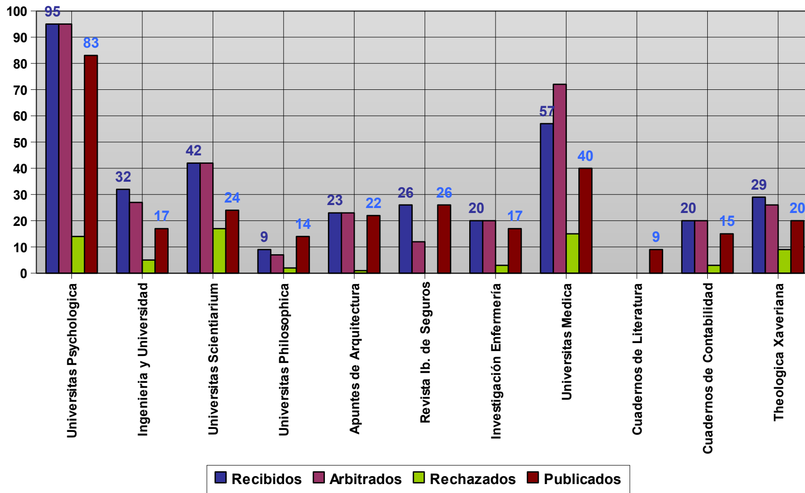
Tratamiento de Artículos por Revista: Recibidos vs. Publicados
