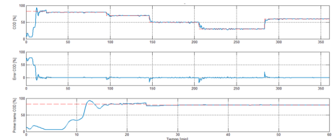
Figura 14. Respuesta de la concentración de oxígeno disuelto en el cultivo.
