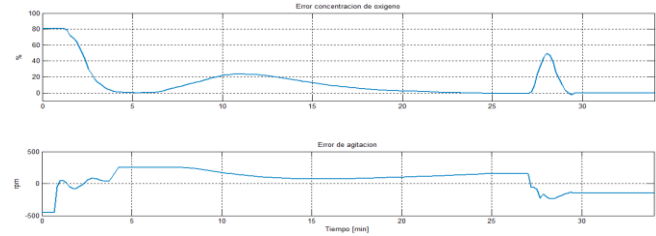
Figura 13. Errores del controlador en agua destilada.
