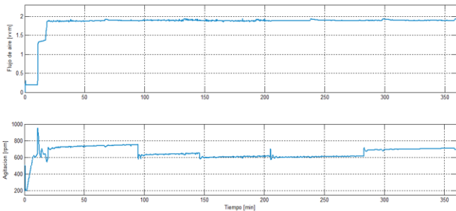
Figura 17. Variables de control en el cultivo.
