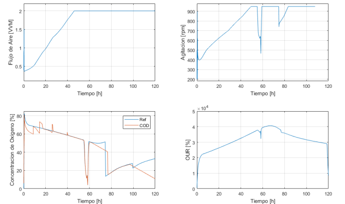
Figura 10. Respuesta del controlador MPC.
