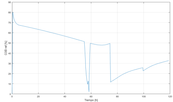
Figura 2. Curva óptima de COD para maximizar la proteína.
