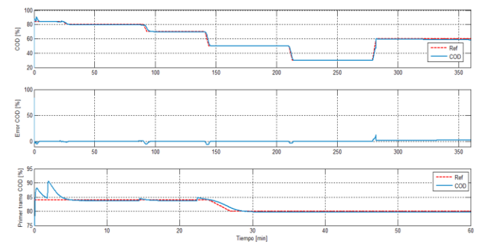
Figura 15. Respuesta de la concentración de oxígeno disuelto en simulación.
