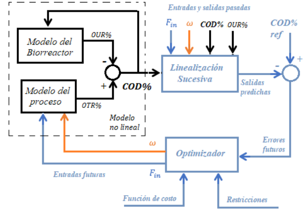
Figura 9. Esquema de control del MPC.
