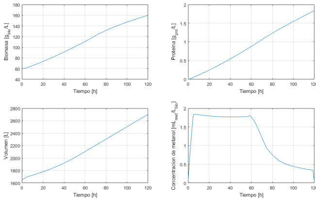
Figura 8. Respuesta del crecimiento de biomasa y proteína.
