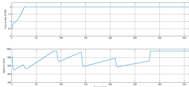
Figura 18. Variables de control en simulación.
