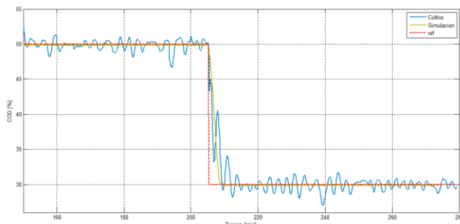
Figura 16. Respuesta de la concentración de oxígeno disuelto en simulación.
