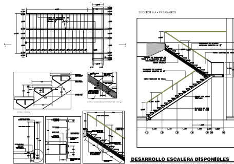
DESARROLLO ESCALERA DISPONIBLES CENTRO INTERACTUANTE DE ARTE CONTEMPORANEO Y TECNOLOGIA
