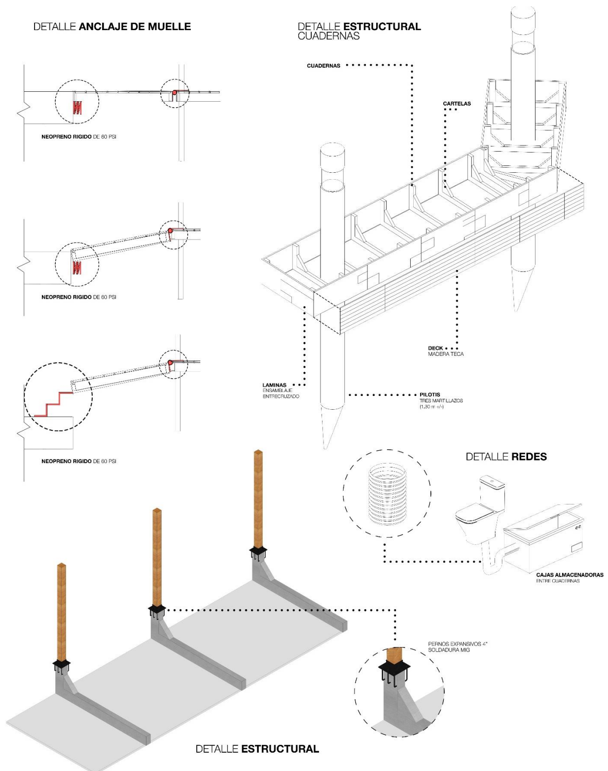
Ilustración 44. Detalles estructurales. Fuente: Elaboración propia
