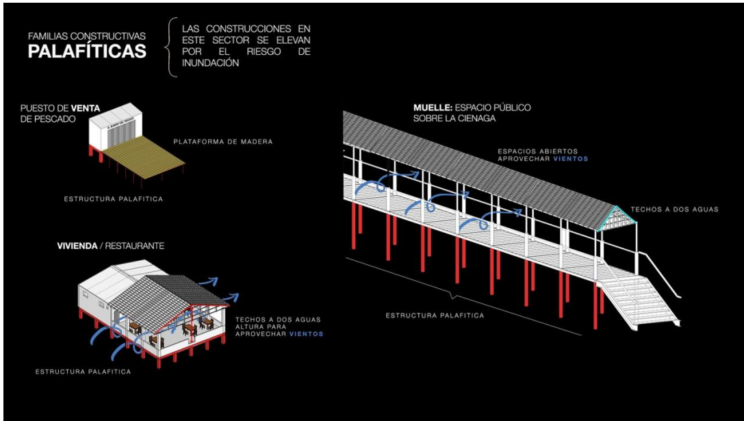
Ilustración 18. Familias constructivas del sector a tratar. Fuente: Elaboración propia
