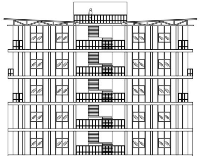
Fachada Lateral E:1:125
