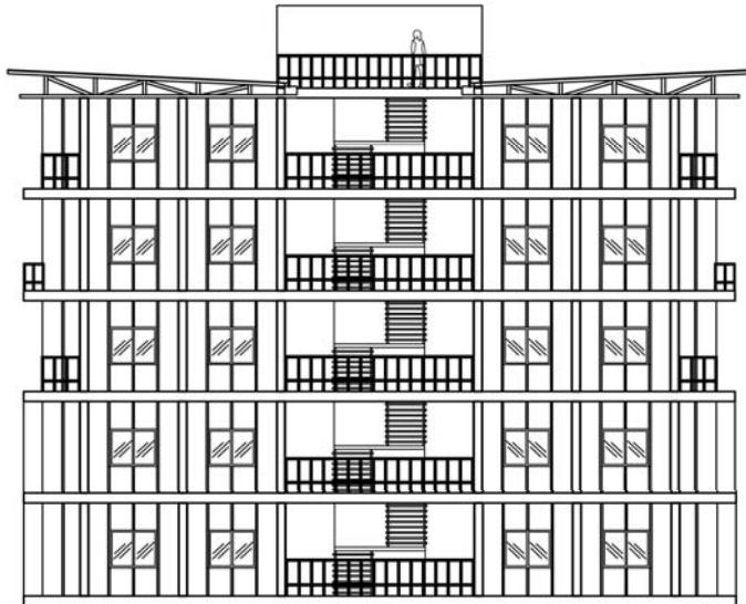
Fachada Lateral E:1:125
