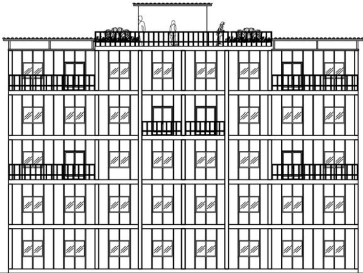
- Fachada Exterior E:1:125
