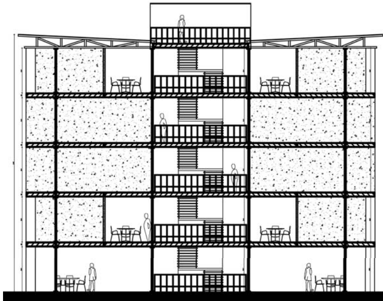
Corte A:A'' E:1:125
